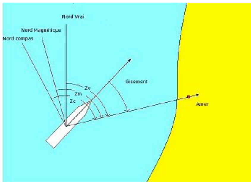
Σχεδιάγραμμα διαφόρων διοπτεύσεων του σημείου Amer.
